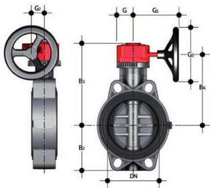
Дисковый затвор ПВХ FEOVRM с редуктором, EPDM, FIP d140 (DN125)
