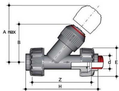
Угловой обратный клапан VR с муфтовыми окончаниями (уплотнение EPDM) PP-H d32 (DN25)
