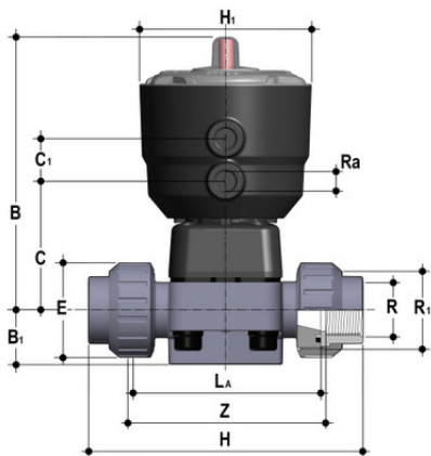
Мембранный клапан ПВХ с пневмоприводом, PN10, DK, EPDM, FIP R1" (DN25)
