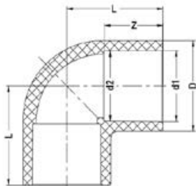
Отвод 90° ХПВХ IPS (Model B) d500 PN10
