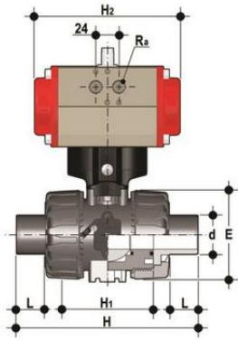
Шаровой кран VKDDVNC ПВХ с пневмоприводом НЗ с втулочными окончаниями, FKM, FIP d63 (DN50)
