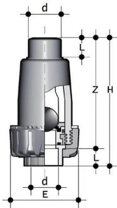
Шаровой обратный клапан SR ПВДФ, муфтовые окончания d32 (DN25)
