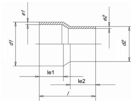
Муфта редукционная ПВДФ (Simona) 110x90 SDR33 PN10
