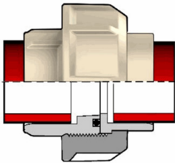
Муфта разборная ПВХ d20 SDR21 PN16
