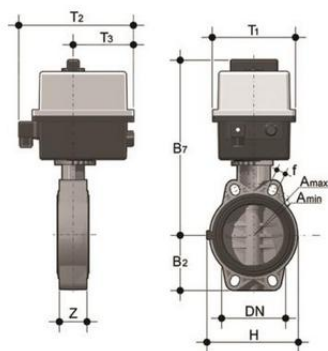
Дисковый затвор общего применения FE ПВХ с эл.приводом 24V AC/DC, FKM, FIP d160 (DN150)
