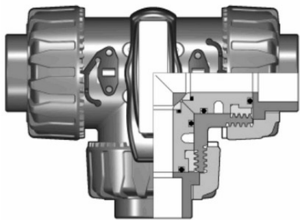
3-х ходовой шаровой кран ПВХ ТКД с муфтовыми окончаниями, Т-шар, FKM, FIP d50 (DN40)
