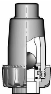
Шаровой обратный клапан SR с муфтовыми окончаниями (уплотнение FKM) PP-H d20
