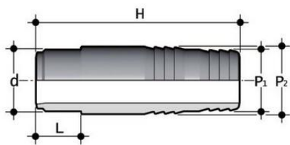
Шланговый адаптер PP-H FIP d50 PN10
