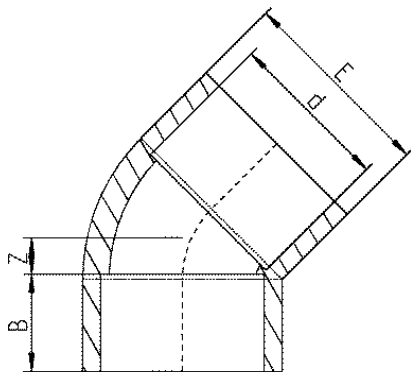
Отвод клеевой 45° PBX Praher Plastics d225
