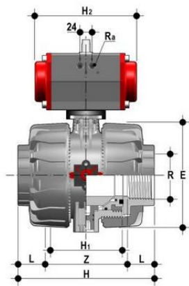
Шаровой кран VKD ПВХ с пневмоприводом НЗ с резьбовыми окончаниями, EPDM, FIP R2 1/2" (DN65)
