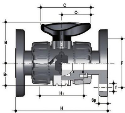
Шаровой кран промышленного применения VKD с фланцевыми окочаниями (уплотнение FKM) PP-H d32
