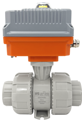
Шаровой кран IVKD ПП-гомополимер с эл.приводом 24V DC, муфтовые окончания, FKM, IPS d50 (DN40)
