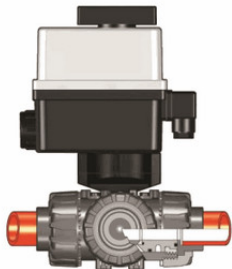
3-х ходовой шаровой кран TKD с эл.приводом 90-240V, муфтовые окончания, Т-шар (уплотнение EPDM) PP-H d40 (DN32)
