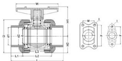
Кран шаровый ХПВХ муфтовый промышленный EPDM IPS d110 (DN90)
