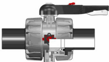
Шаровой кран промышленного применения VKD с патрубками из ПЭ (CVDE) (уплотнение FKM) PP-H d110 (DN100)
