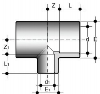
Редукционный тройник ХПВХ 50х25 PN16
