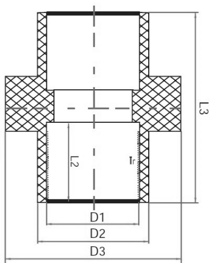
Муфта разборная с ВР ПВХ IPS 20x1/2"
