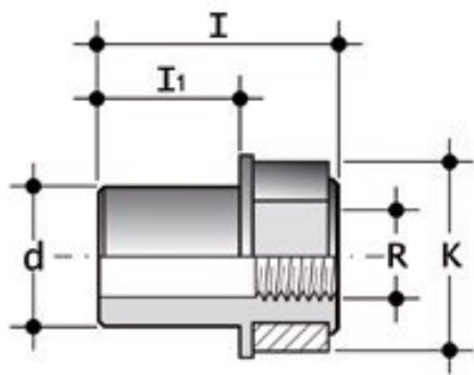
Адаптер с внутренней резьбой PP-H FIP 25x3/4 SDR11 PN10
