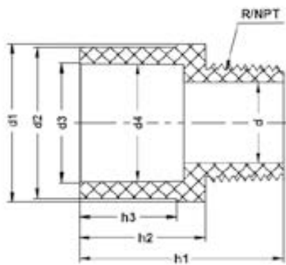
Редукционная муфта ПВДФ с НР для раструбной сварки 32x1" PN 16
