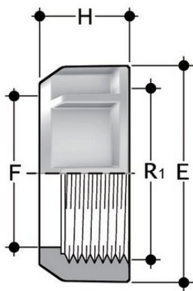
Гайка ПВДФ d1 SDR21 PN16
