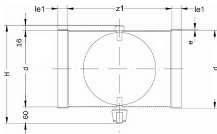
Дроссельный клапан со ступенчатой регулировкой PPs d110
