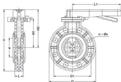
Затвор дисковый ПВХ с рукояткой общего применения EPDM IPS 63 (DN50)
