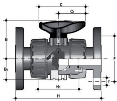
Шаровой кран промышленного применения VKD ХПВХ с фланцевыми окончаниями d32 (DN25)
