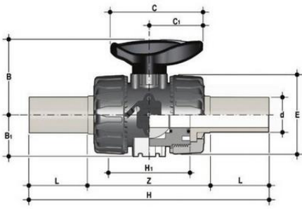
Шаровой кран VKD ПВДФ с длинными патрубками d32 (DN25)
