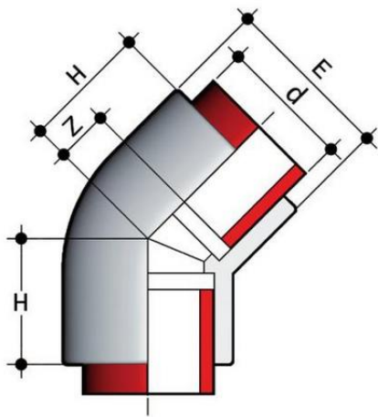
Отвод ПВДФ 45° d50 SDR21 PN16
