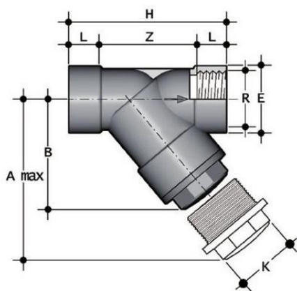
Грязевый фильтр из серого ПВХ с резьбовыми окончаниями, EPDM, FIP R4" (DN100)
