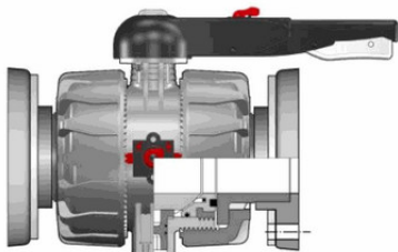
Шаровой кран промышленного применения VKD С фланцевыми окончаниями (уплотнение FKM) PP-H d90
