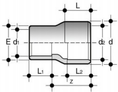
Втулка редукционная ПВХ FIP (трехразмерная) 32x25x25
