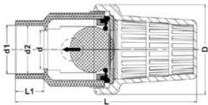
Донный клапан IVZ ПВХ с муфтовыми окончаниями, FKM, FIP d40 (DN32)
