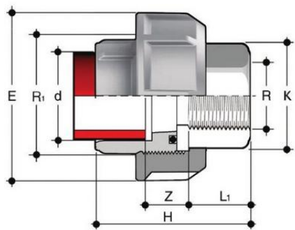
Муфта разборная переходная PP-H / нерж.сталь, ВР (EPDM) FIP 50x1 1/2 PN10
