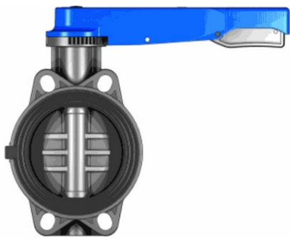
Дисковый затвор ПВХ FEOVLM с рукояткой, FKM, FIP d225 (DN200)
