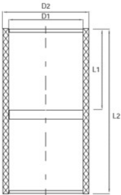
Муфта соединительная ХПВХ IPS (Model A) d110 PN16
