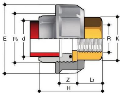
Муфта разборная переходная РР-Н / латунь, ВР (EPDM) FIP 63x2 PN10
