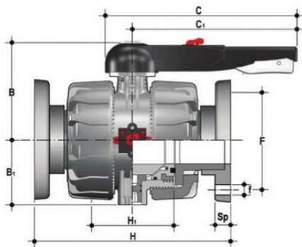
Шаровой кран промышленного применения VKD С фланцевыми окончаниями (уплотнение FKM) PP-H d75 (DN65)
