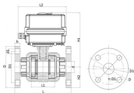
Шаровой кран IVKD PBX с эл.приводом 220V AC, фланцевые окончания, FKM, IPS d90 (DN80)
