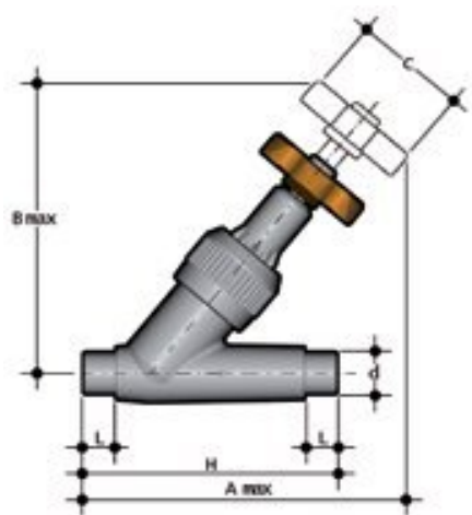
Угловой вентиль VVDV ПВХ с втулочными окончаниями, EPDM, FIP d40 (DN32)
