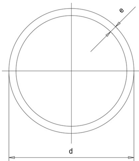
Труба ПВДФ (Simona) d125 SDR33 PN10
