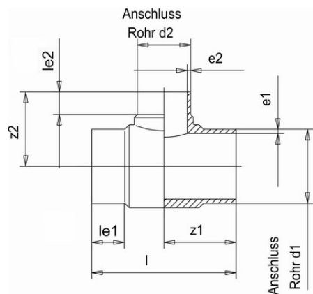
Тройник редукционный PP-H Simona (PN6) 140x63 SDR17.6 PN6
