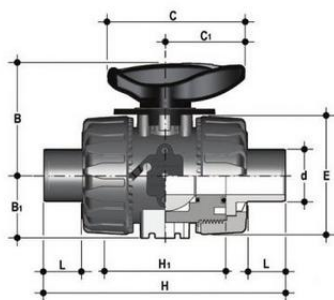
Шаровой кран ПВХ для регулирования потока VKR со втулочными окончаниями, FKM, FIP d16 (DN10)
