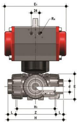
3-х ходовой шаровой кран ТКД ПБХ с пневмоприводом ДвД с муфтовыми окончаниями, Т-шар, FIP d20 (DN15)
