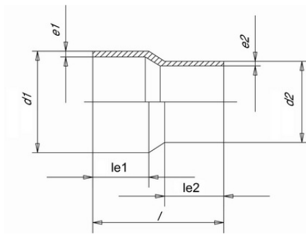
Муфта редукционная ПВДФ (Simona) 50х40 SDR21 PN16
