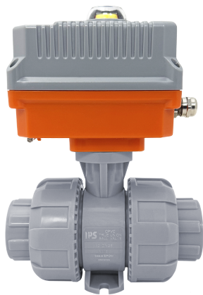
Шаровой кран IVKD ХПВХ с эл.приводом 24V DC, муфтовые окончания d40 (DN32)
