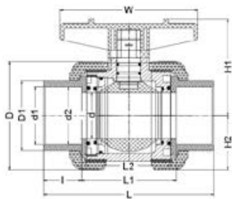
Кран шаровой промышленного применения с муфтовыми окончаниями PP-H IPS d110
