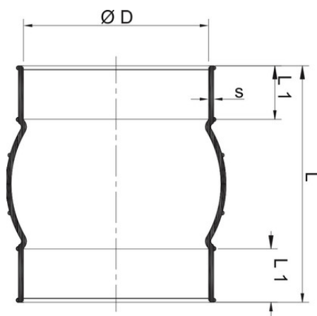
Шаровая манжета с лентой PPs d315
