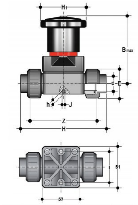
Компактный мембранный клапан CM ПВХ с пневмоприводом НЗ, резьбовые окончания, FKM, FIP 3/8"
