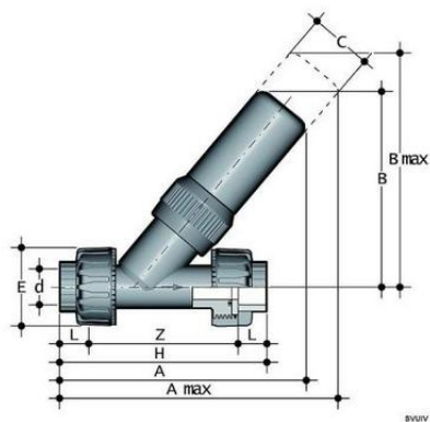
Угловой предохранительный клапан SV PBX с муфтовыми окончаниями, FKM, FIP d25 (DN25)
